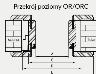
D - wymagana szerokość otworu w murze
