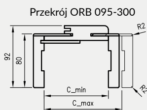
Przekrój ORB 095-300
