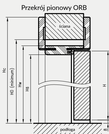
Przekrój pionowy ORB
