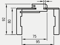
Przekrój ORB 095-300
