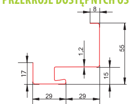
Ościeżnica stalowa z uszczelką do drzwi stalowych technicznych 40 FD-21/N
