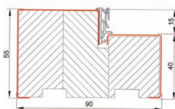
Ciepła ościeżnica stalowo-drewniana z uszczelką do drzwi stalowych zewnętrznych 55, 55 LUX, 72 LUX, 72 LUX TERMO
