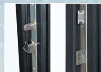
Zamek hakowo-bolcowy ROTO z cichą zapadką
