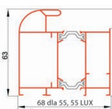
Ciepła ościeżnica aluminiowa z uszczelką do drzwi stalowych zewnętrznych 55, 55 LUX, 72 LUX, 72 LUX TERMO
